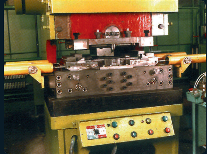
Przyrząd typu TRD Device type TRD
