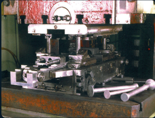
Przyrząd typu TRL Device type TRL
