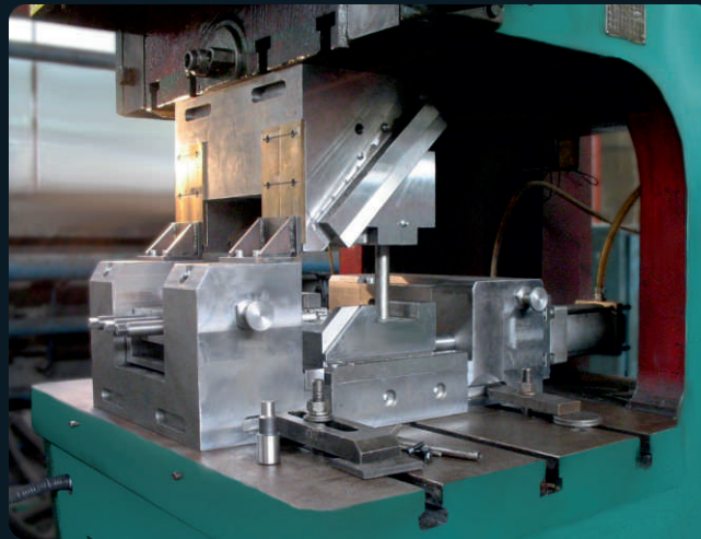
Przyrząd typu PKJ Device type PKJ
